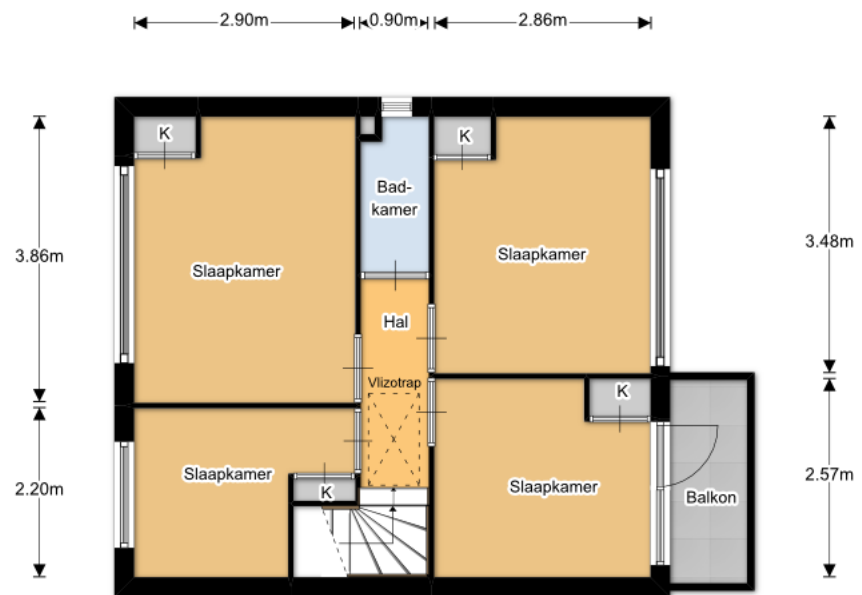
1e Verdieping
